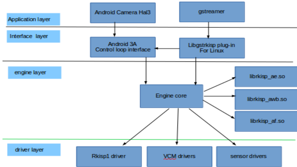
图 2.1-1 camera engine 模块结构
