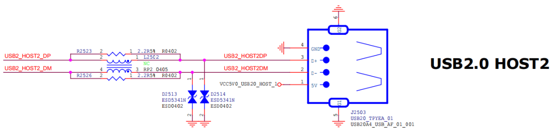
图 2-16 RK356x USB 2.0 Host 接口
