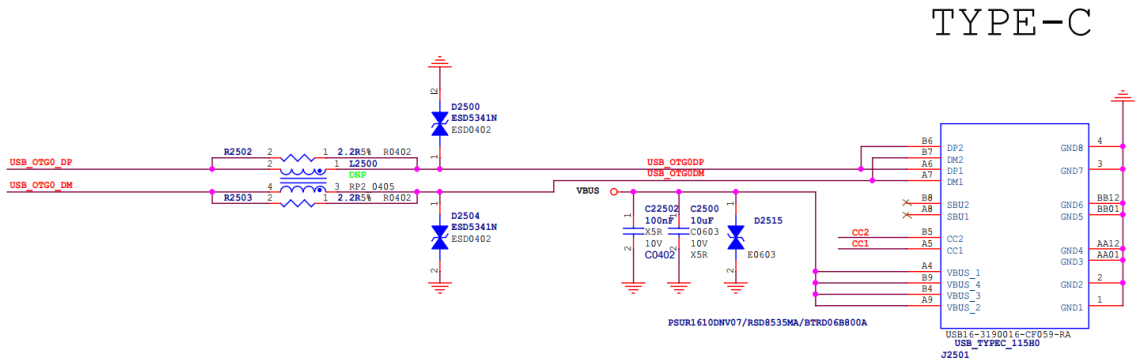
图 2-10 RK3566 USB 2.0 OTG Type-C 接口
